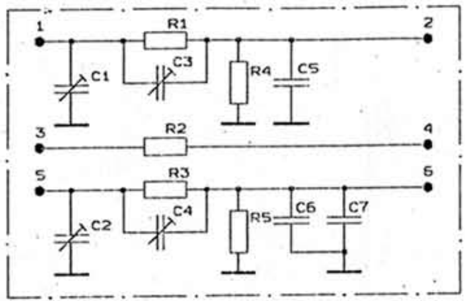
Схема плат А1, А2
