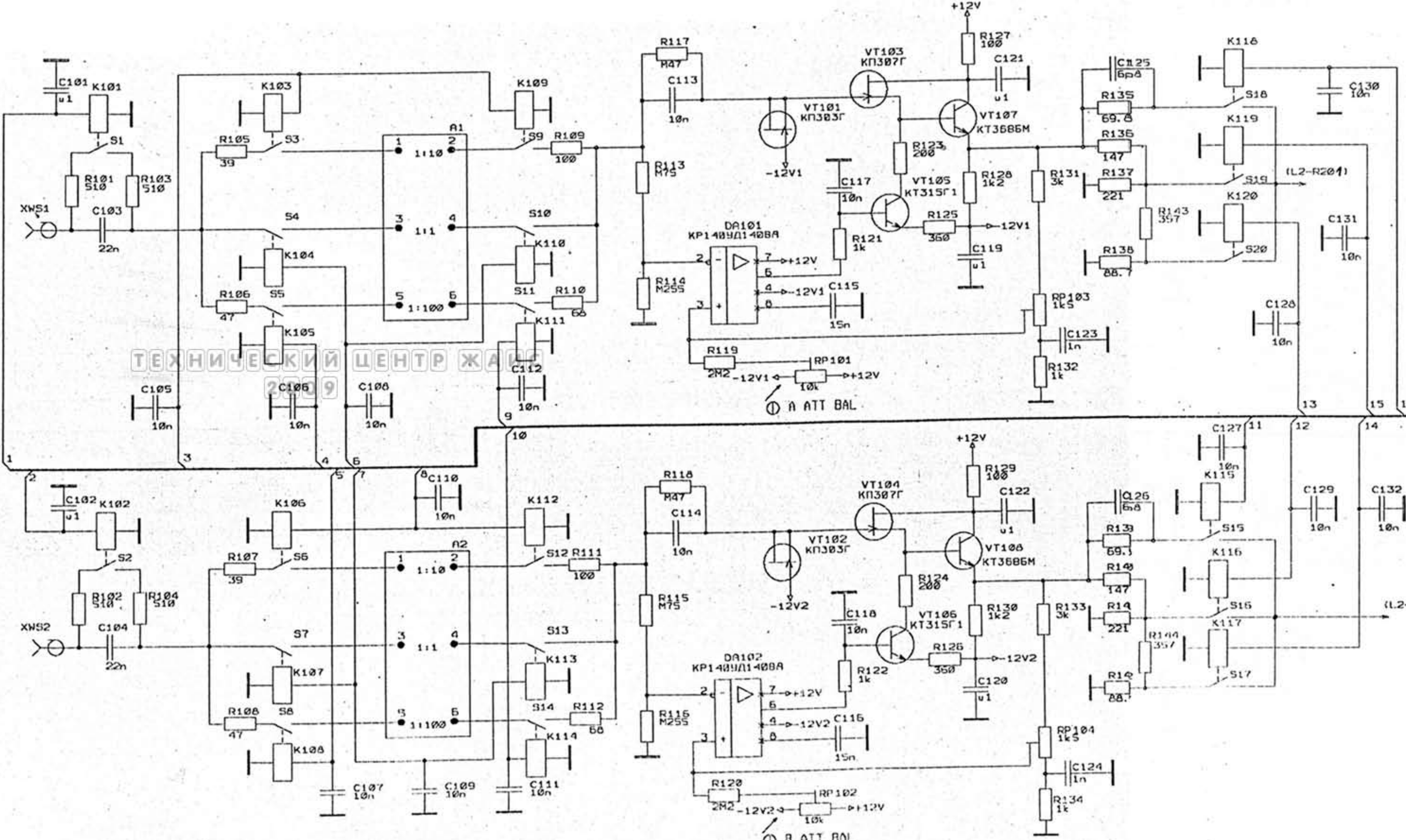
Схема плат А1, А2
