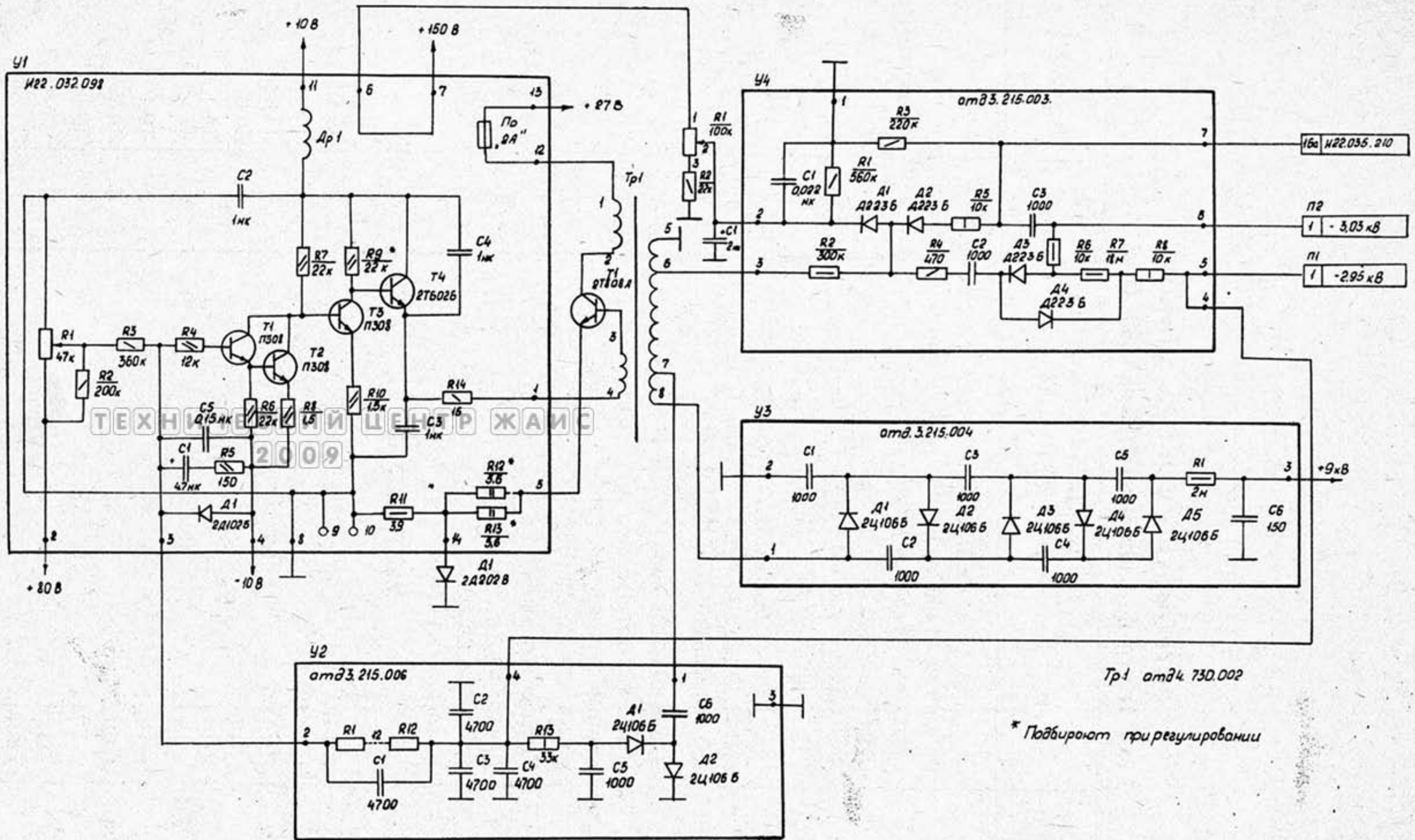
Осциллограф универсальный С1-78 ПРЕОБРАЗОВАТЕЛЬ ВЫСОКОВОЛЬТНЫЙ Схема электрическая принципиальная И23.211.028 33
