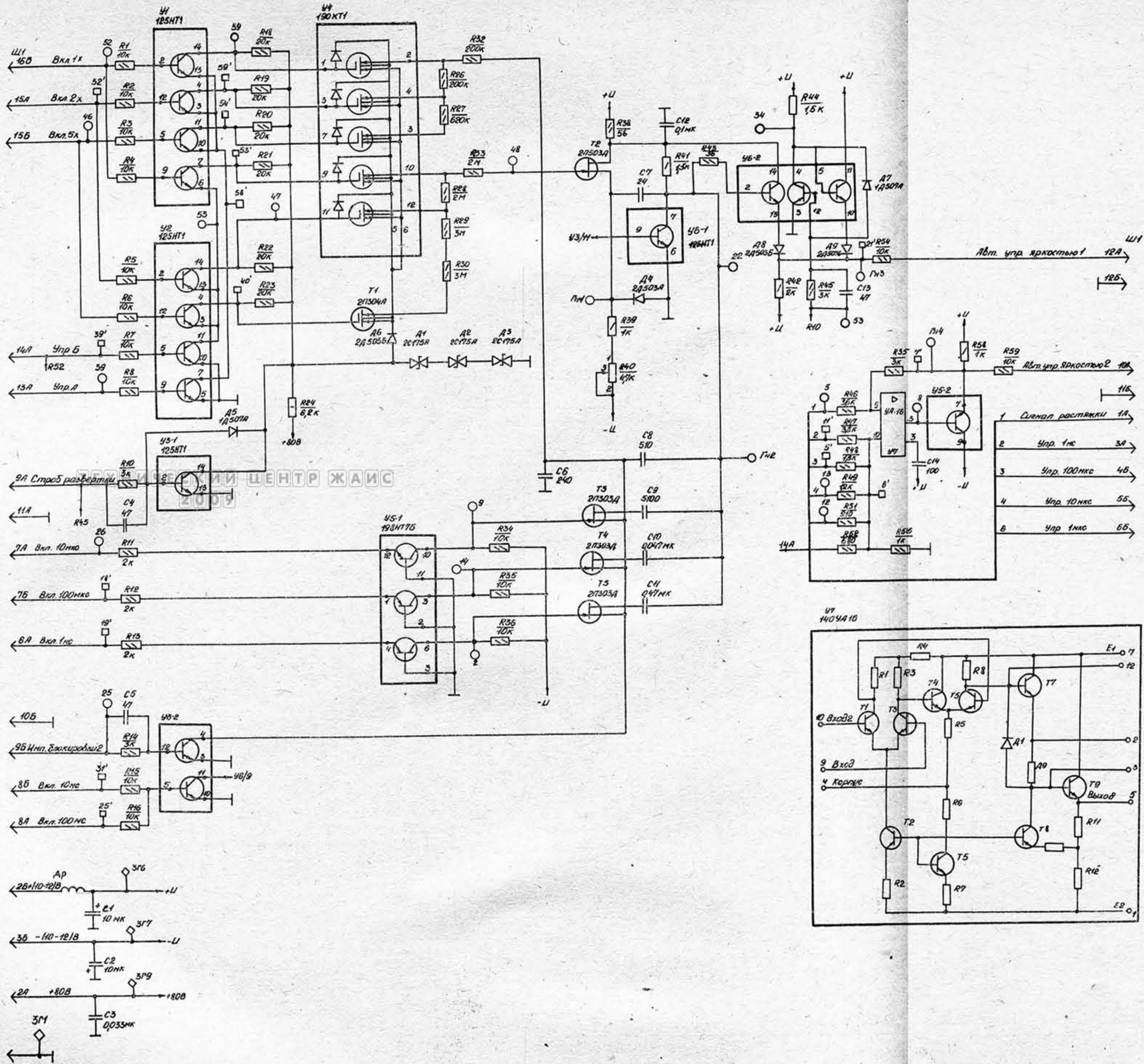
Осциллограф универсальный С1-78 АВТОМАТИКА Z Схема электрическая принципиальная И22.070.122 Э3
