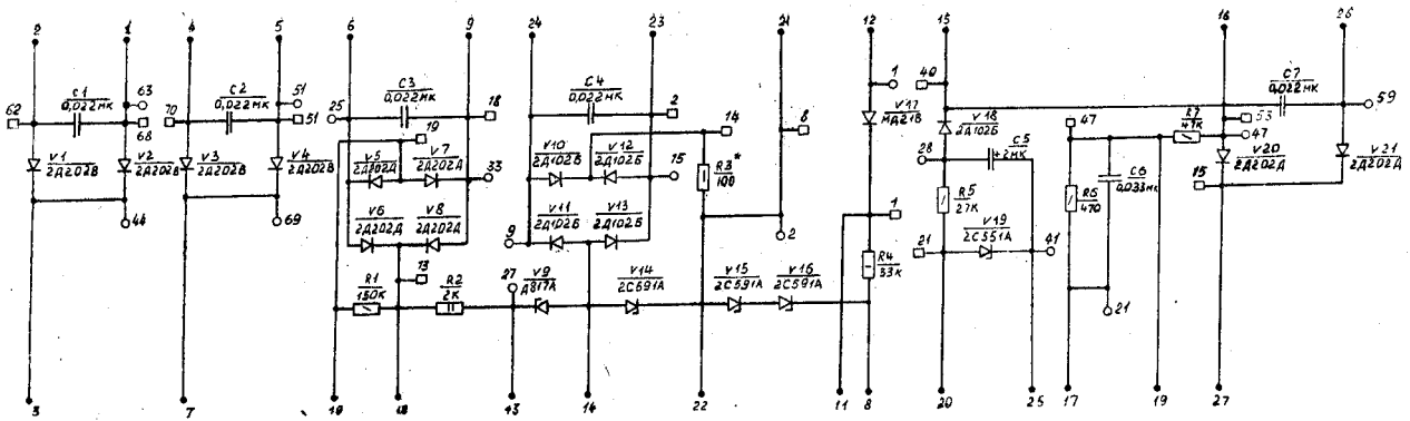
ВЫПРЯМИТЕЛЬ Схема электрическая принципиальная И23.215.189ПЭ3
