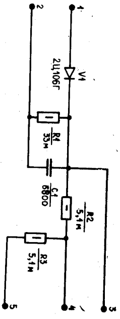
Выпрямитель Схема электрическая принципиальная ИЭ3.215.16793
