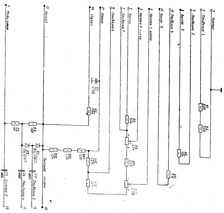
Выпрямитель Схема электрическая принципиальная ИЭ3.215.16793
