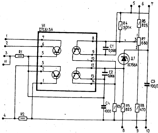
СТАБИЛИЗАТОР Схема электрическая принципиальная И23.233.122Э3
